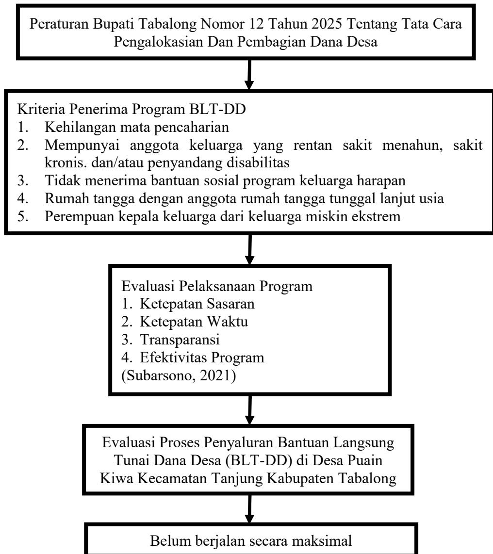
Gambar 1 Kerangka Konseptual
